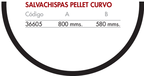
Curvatura del savachispas circular
