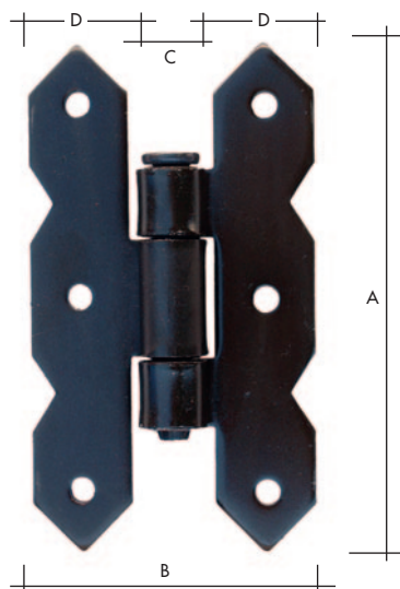
BISAGRA MODELO MARIPOSA
